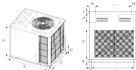
Modelo: GK-H15NH3AF
