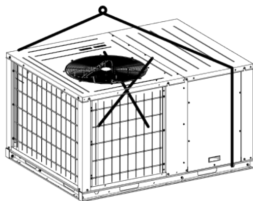
Incorrecto
