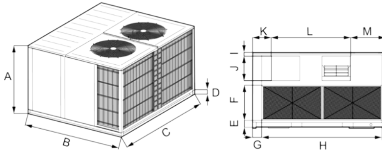
Modelo: GK-H20NH3AF
