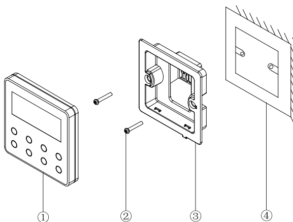
Fig. 7.23 Componentes del controlador de zona
